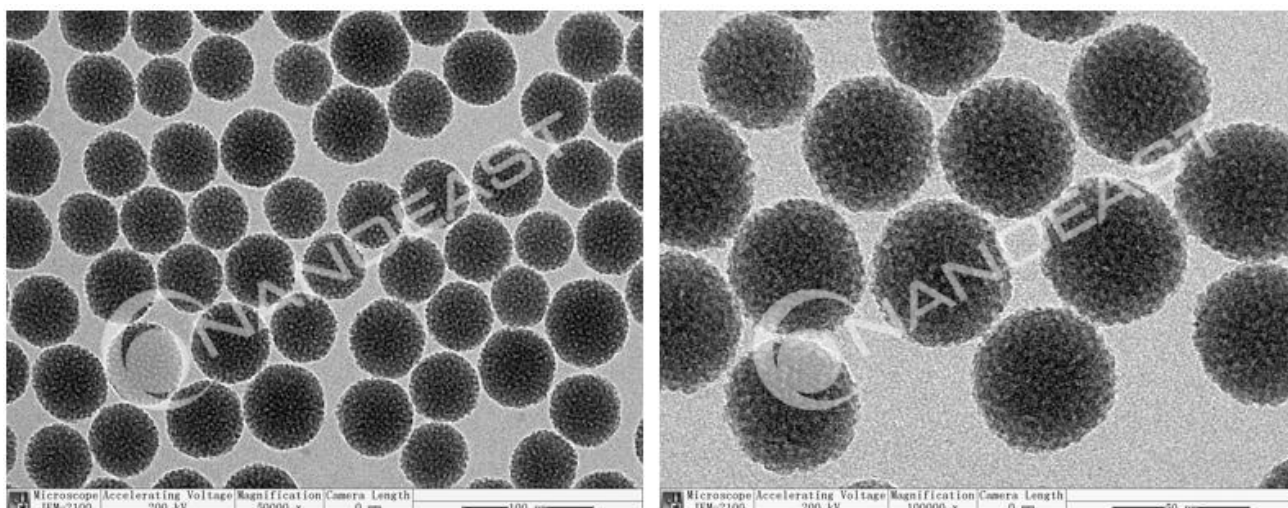
图: 50nm 介孔二氧化硅纳米颗粒的透射电镜图片
