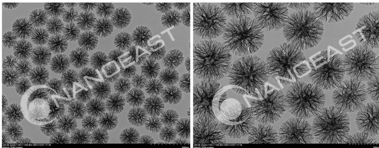
图: 200nm 树枝状介孔二氧化硅纳米颗粒的透射电镜图片
