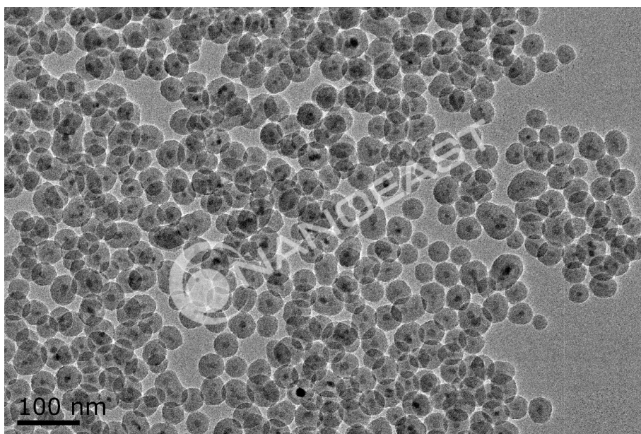
图 1 核壳结构的 \text{SiO}_2@\text{Fe}_3\text{O}_4 纳米颗粒的透射电镜图
