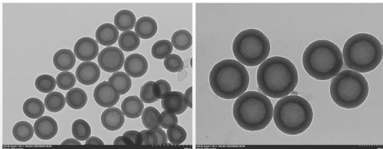
图: 350 nm 中空介孔二氧化硅纳米颗粒的透射电镜图片
