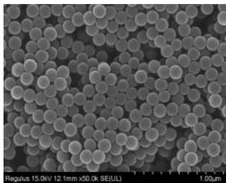
图 1. 120 nm 聚苯乙烯微球的扫描电镜图
