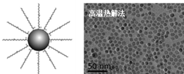
图 1. 10 nm 油酸修饰的四氧化三铁磁性纳米颗粒示意图和 TEM 照片 油酸修饰的四氧化三铁磁性纳米颗粒 (OA@Fe 3 O 4 , 高温热解法)
